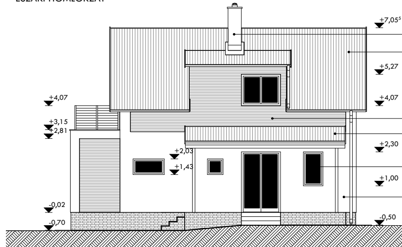
ÉSZAKI HOMLOKZAT
