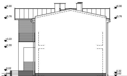
DÉL-KELETI HOMLOKZAT
