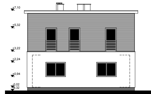
ÉSZAK-NYUGATI HOMLOKZAT
